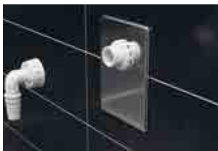
8. Inox poklopac postaviti, i pomoću navojne matice pričvrstiti. Nakon toga priključno koleno, na navoj, ručnom snagom naviti.
